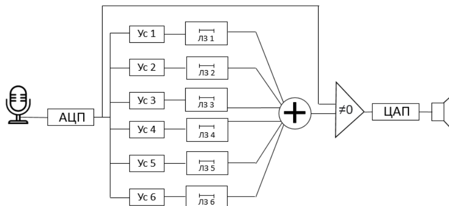
Рисунок 3.4 – Процесс многоканального формирования речеподобной помехи
