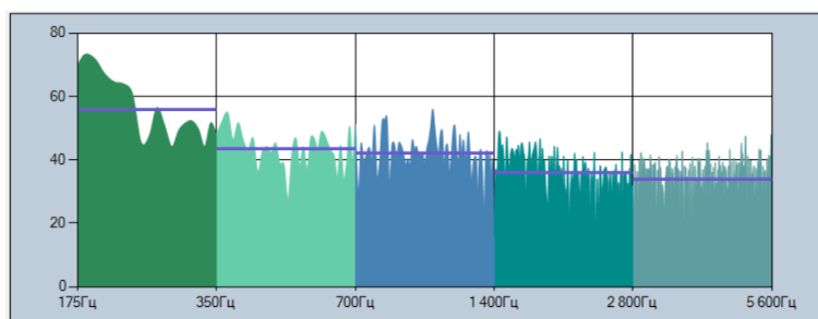
Рисунок 4.9 – Результат применения метода усреднения шума
