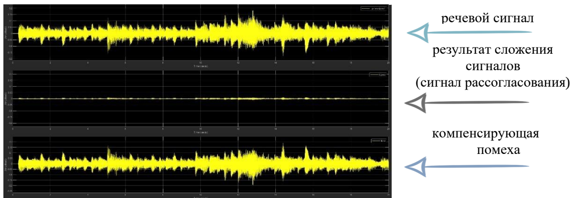
Рисунок 3.14 – Результат моделирования при установке фазы 180 градусов
