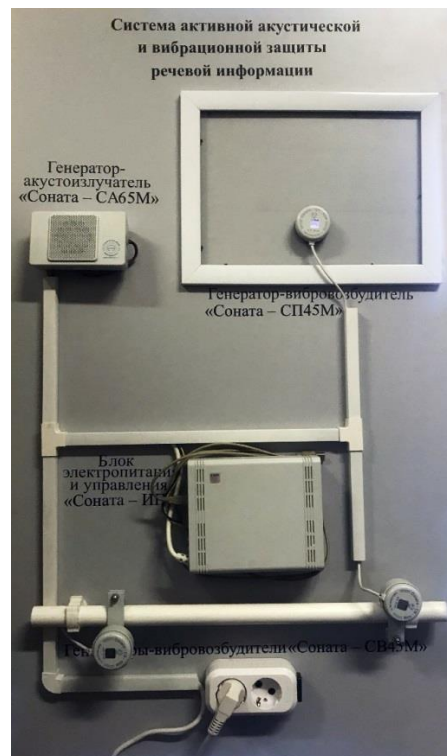
Рисунок 4.7 – Реализованный стенд «Система активной акустической и вибрационной защиты речевой информации»
